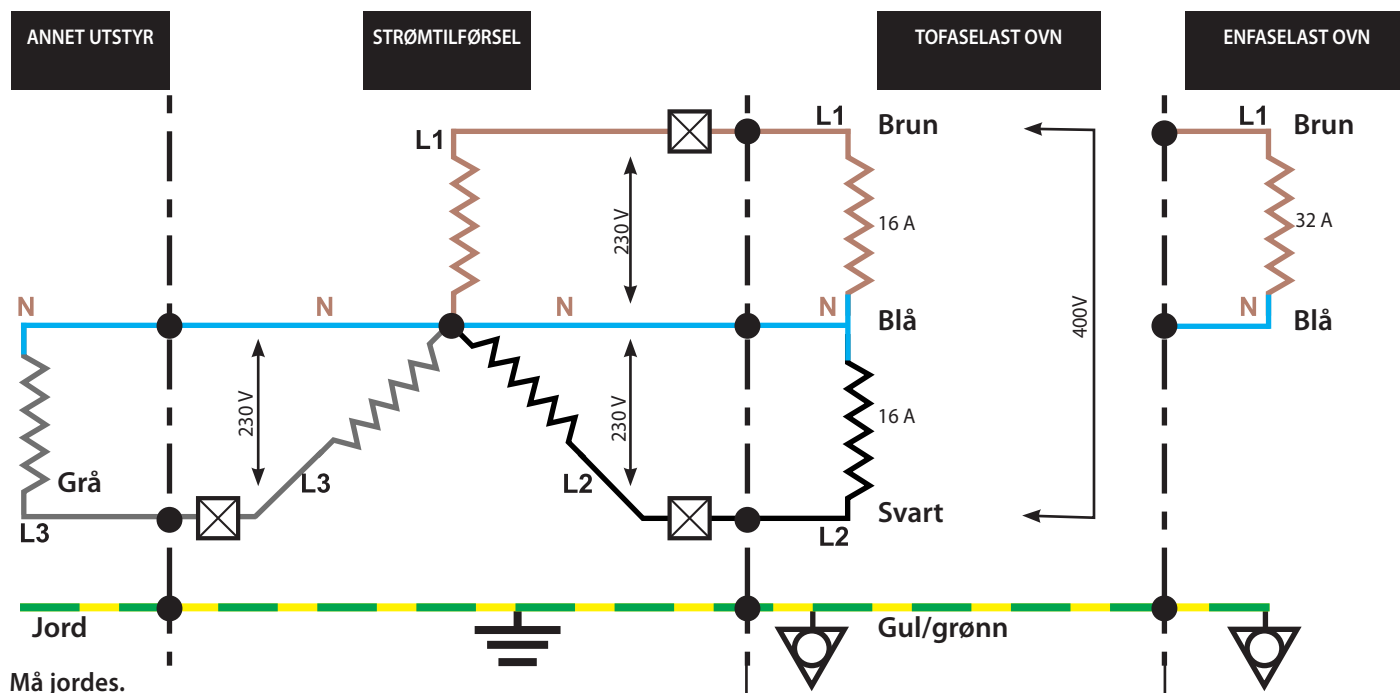
Faselastdiagram
